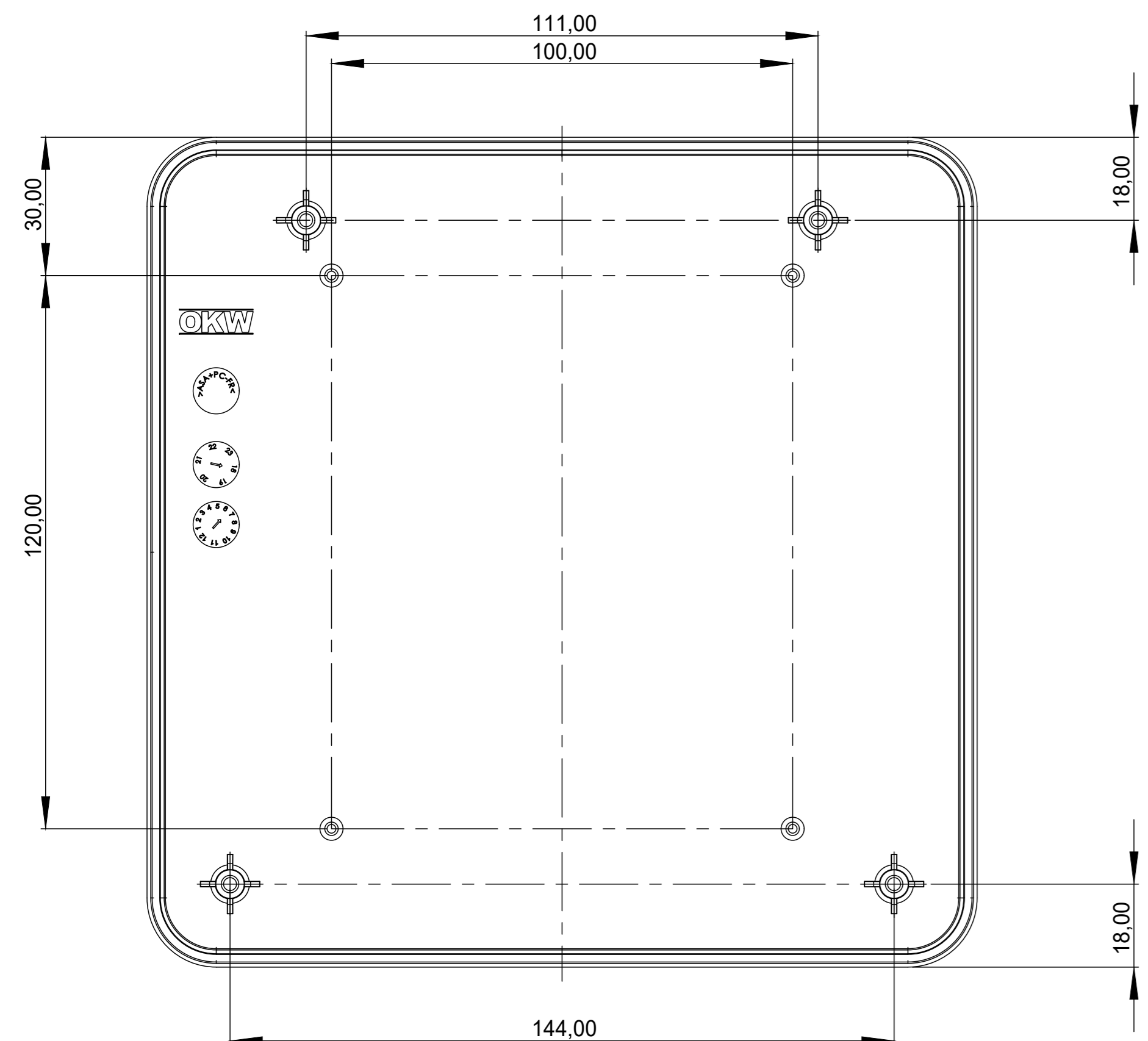
Oberteil Top Part
